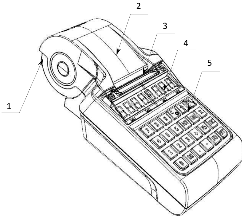
Рисунок 1. Вид спереди/сверху/слева
